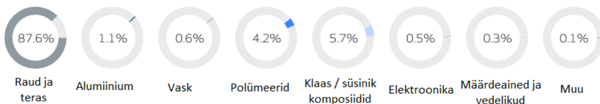
Joonis 57. Tuuliku komponendid (ilma vundamendita). Allikas: https://www.vestas.com/en
