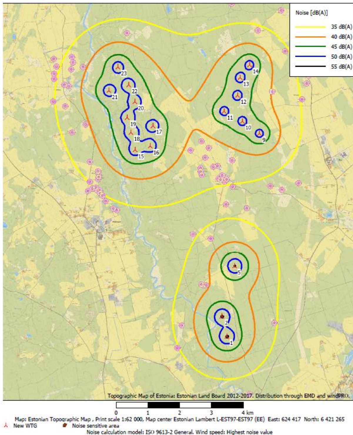
Joonis 59. Mūra leviku kaart 4 m kõrgusel ala 4 tuulikud 107,8 dB +2dB, ala 3 tuulikud 105 dB +2dB ja ala 2 tuulikud 104 dB +2dB.
