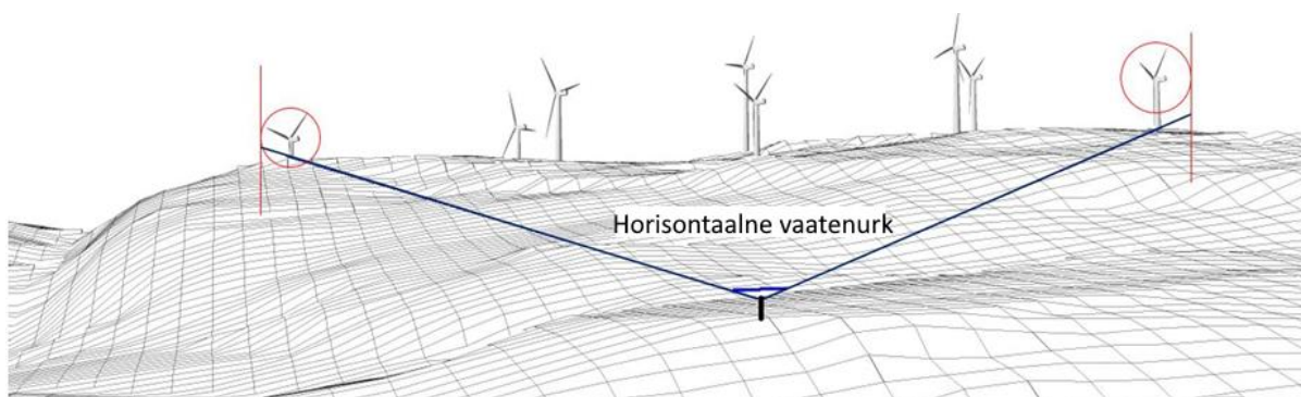
Joonis 69. Horisontaalne vaatenurk. Allikas: WindPro 4.0 kasutusjuhend.
