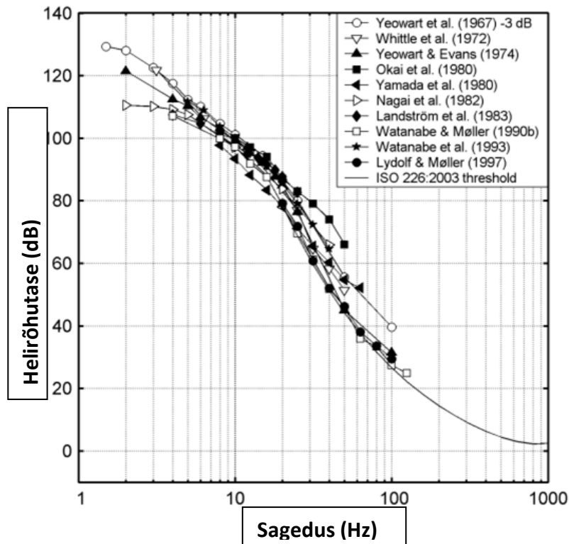
Joonis 60. Inimese heli tajuvus sõltuvana heli sagedusest ja rõhust erinevate teadusuuringute alusel 183 .
