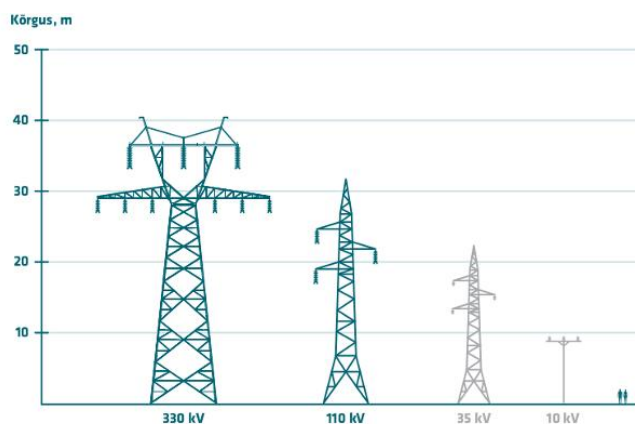
Joonis 79 Erineva pingeklassiga õhuliinide mastid. Allikas: Elering AS.
